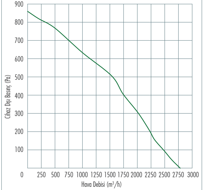
Performans Eğrisi
