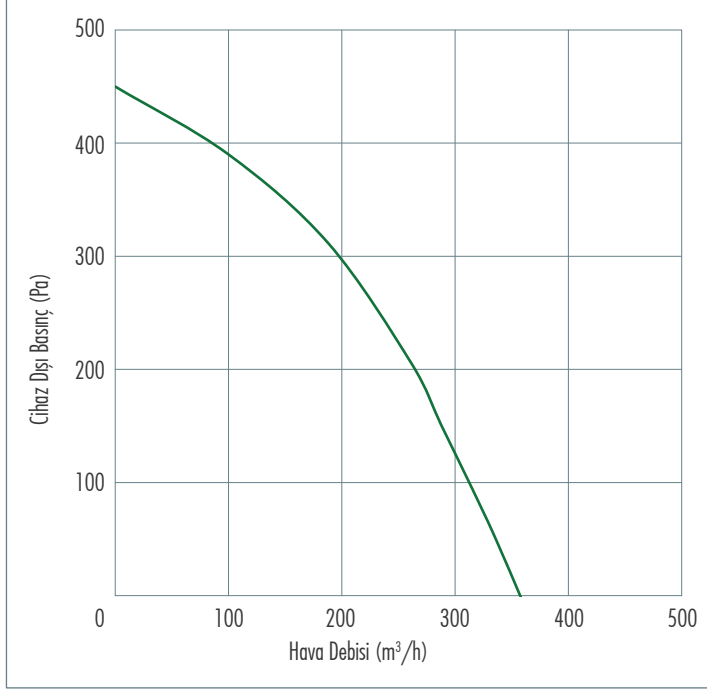
Performans Eğrisi
