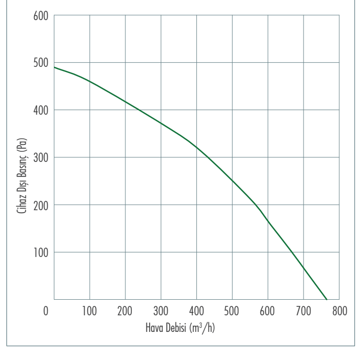
Performans Eğrisi
