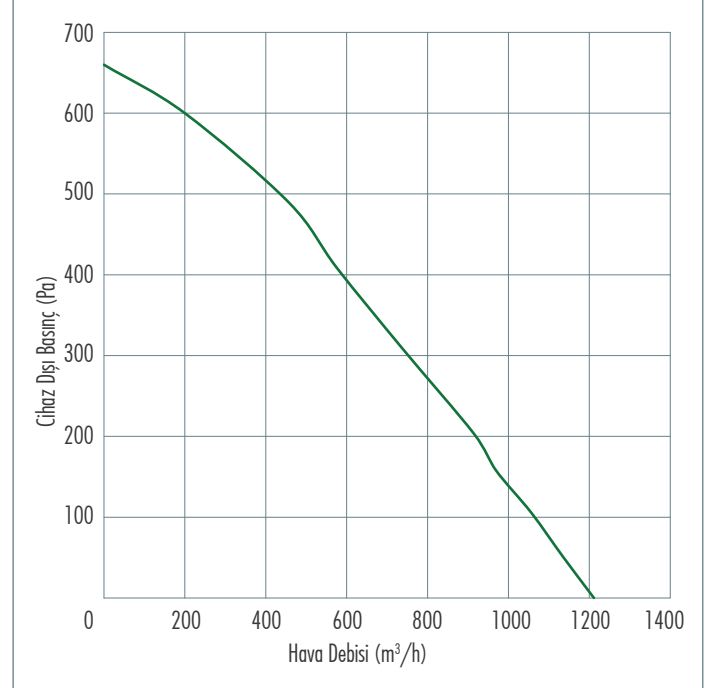
Performans Eğrisi
