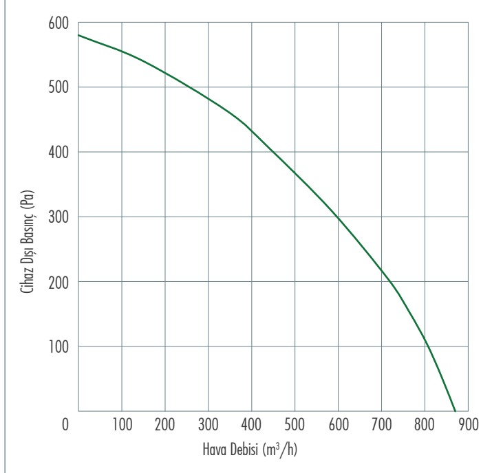
Performans Eğrisi
