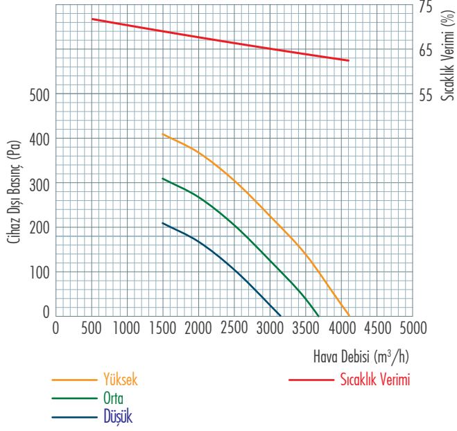
Performans Eğrisi
