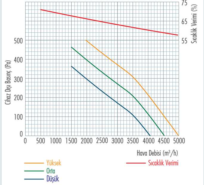
Performans Eğrisi
